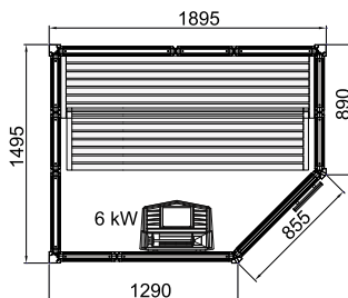
Impression sauna i1915/c 本体価格：3,696,000円
