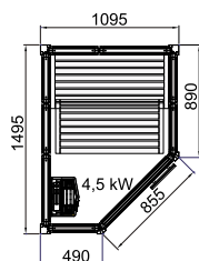
Impression sauna i1115/c 本体価格：2,530,000円
