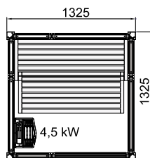
Impression sauna i1313 本体価格：2,640,000円
