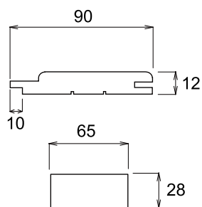
サウナ専用羽目板（アスペン）
