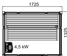
Impression sauna i1713 本体価格：3,168,000円
