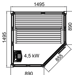
Impression sauna i1515/c 本体価格：2,904,000円
