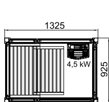
Impression sauna i1309 本体価格：2,508,000円
